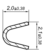
Corte B-B
