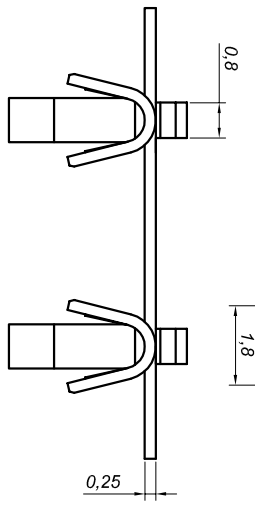
Corte A-A
